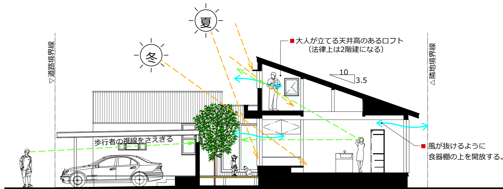
断面図 S = 1 : 100
