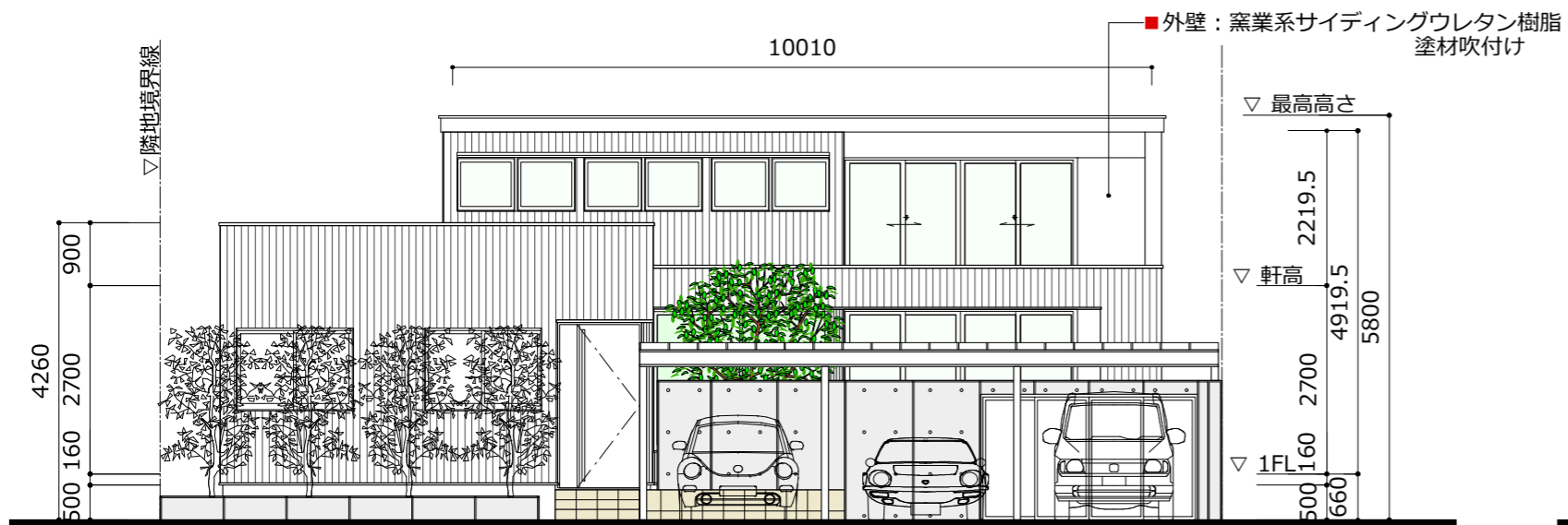
南立面図 S = 1 : 100
