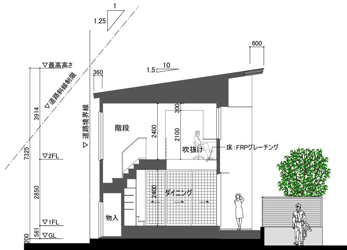
断面図 S=1:100
