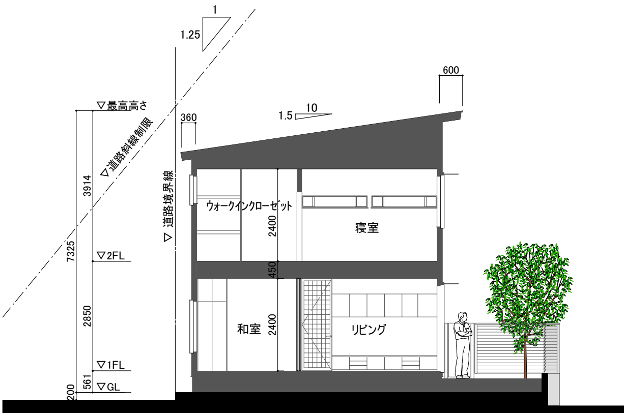
断面図 S=1:100
